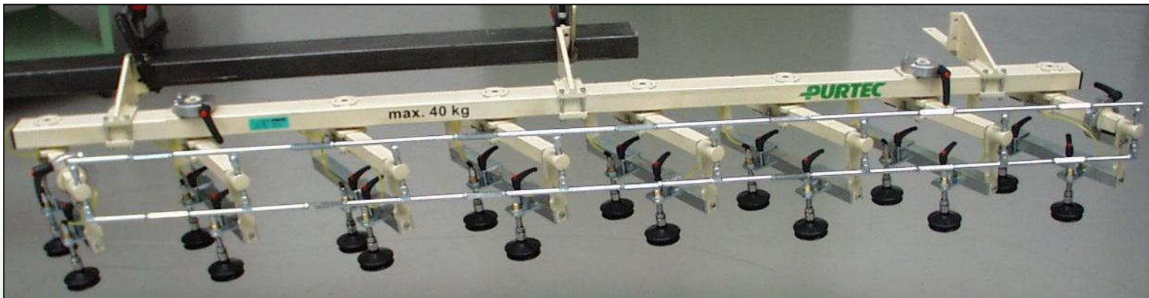
Dachziegelgreifer 8-fach mit Neigungsverstellung
